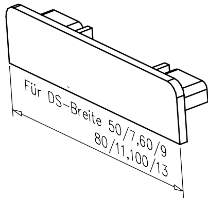
Deckschienenabschluß
