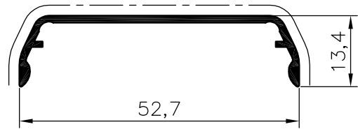
Trapez-Klipsabdeckung 53/13
