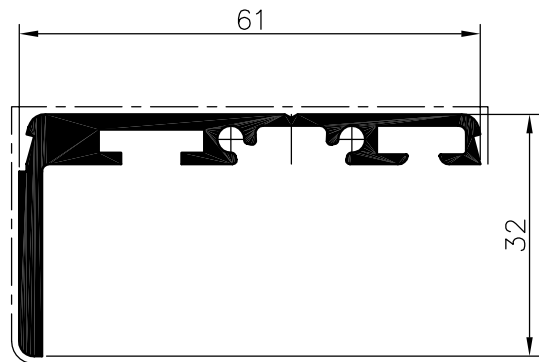
Stirnwanddeckschiene 60/6
