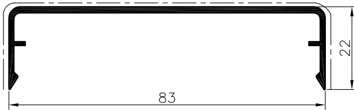
Klipsabdeckung 83/22
