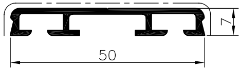
Flachdeckschiene 50/7
