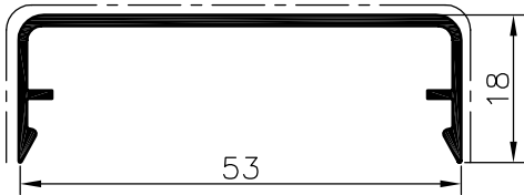
Klipsabdeckung 53/18
