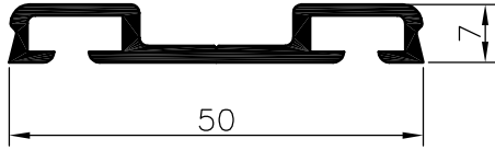
Klipsdeckschiene 50/7
