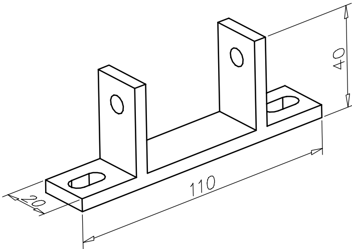
Sprossenschuh
