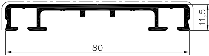
Flachdeckschiene 80/11
