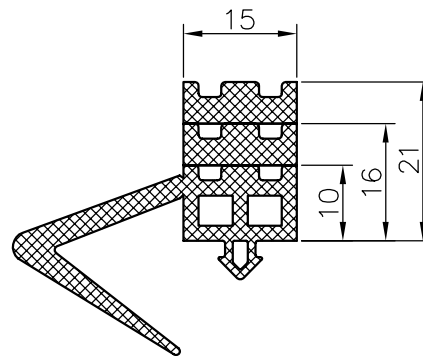
Stirwandabschlussdichtung coex./weiß
