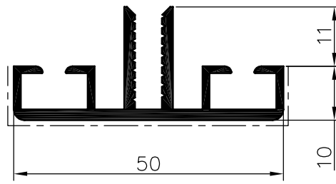
Sprosse 50/10
