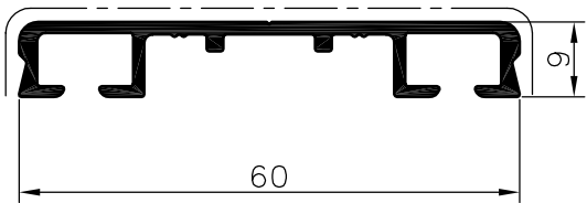
Flachdeckschiene 60/9
