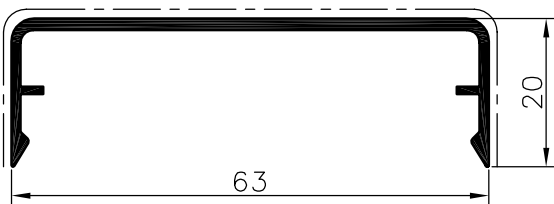
Klipsabdeckung 63/20
