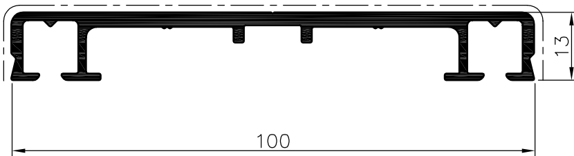
Flachdeckschiene 100/13
